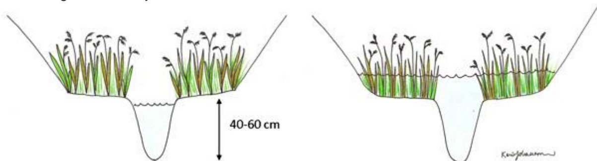
Tvästegsdike vid lågvatten - till vänster - och högvatten - till höger. Illustration: Karin Johansson, Linköpings universitet
